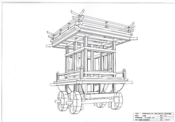
新上川岸区 山車立体図
