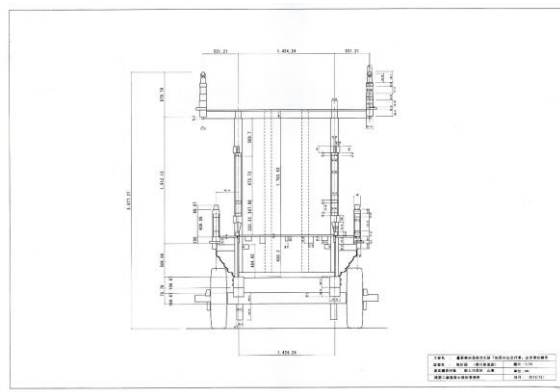
新上川岸区 山車梁行断面図
