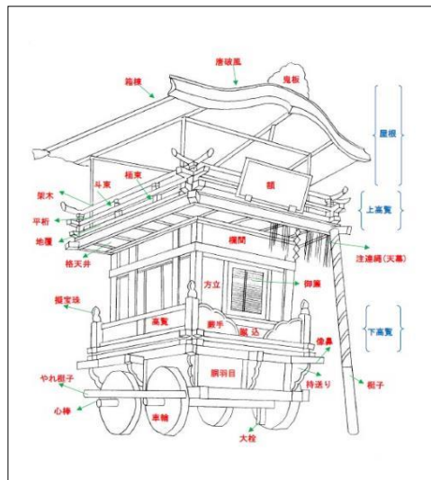
小見川屋台部位図
