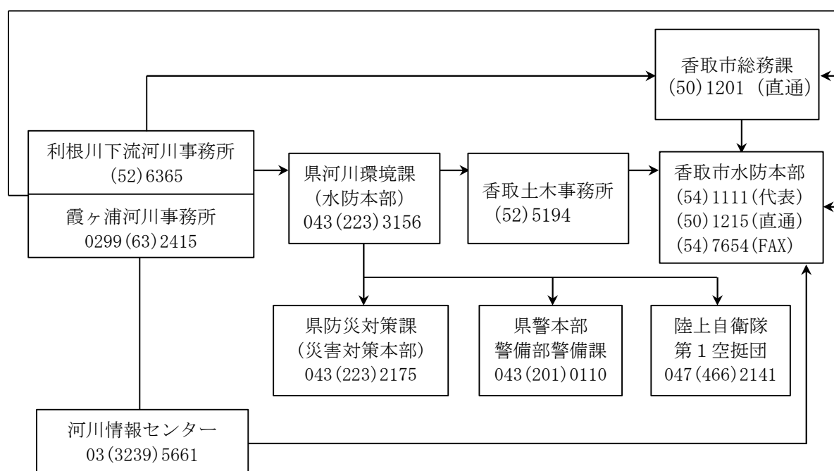
水防警報伝達系統図
