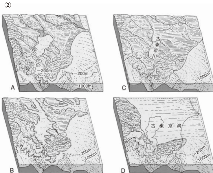
②関東平野の変遷を示す立体古代地図 A.現在 B.縄文前期(約6,000年前) C.最後の氷期の海面最大低下期(約2万年前、先土器時代) D.最後の間氷期の海面最大上昇期(12万年前)
