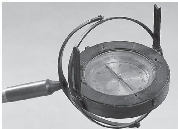
伊能忠敬翁が全国測量をする際に使用した 杖先方位盤(コンパス)
