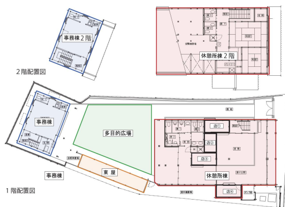
施設配置図
