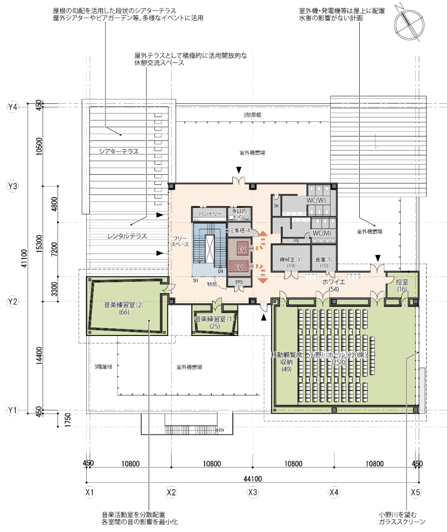
4階平面図
