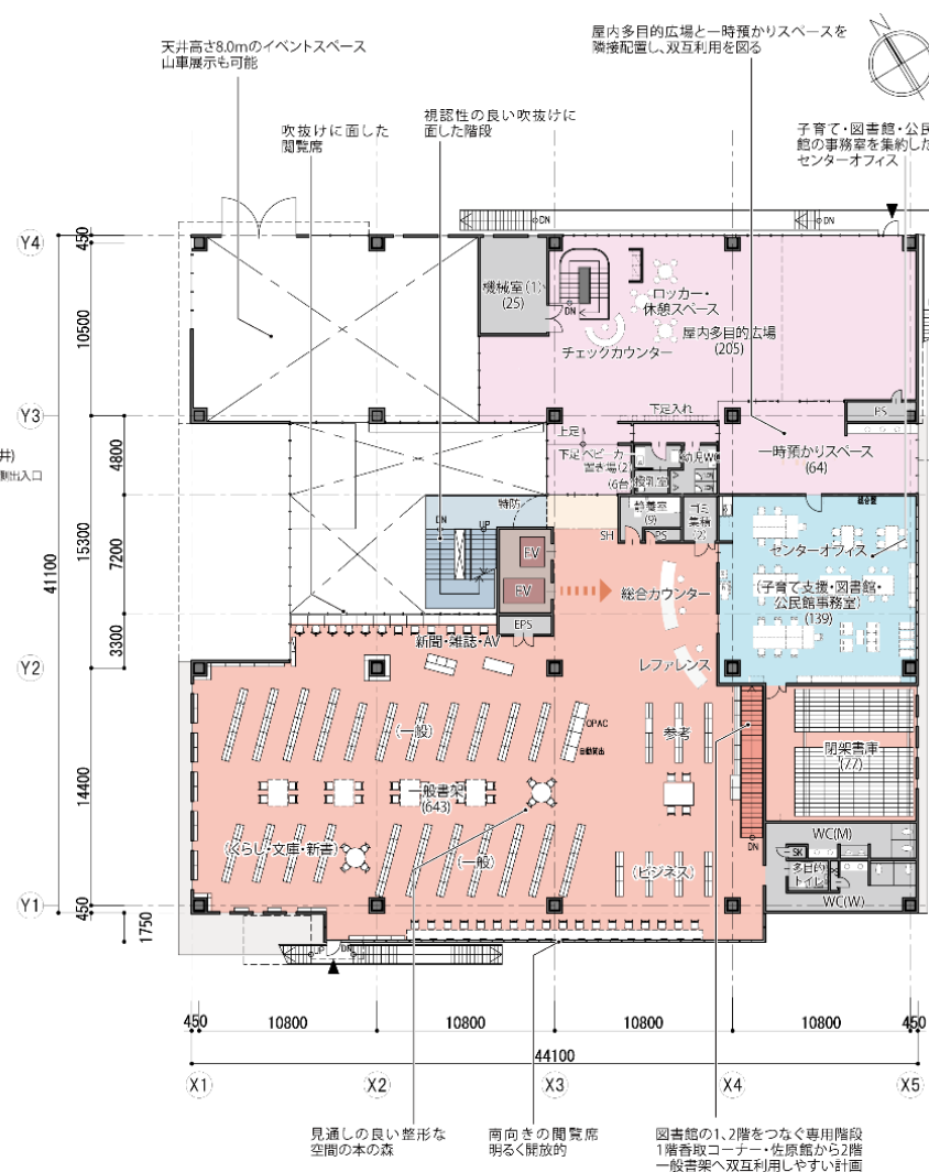
2階平面図
