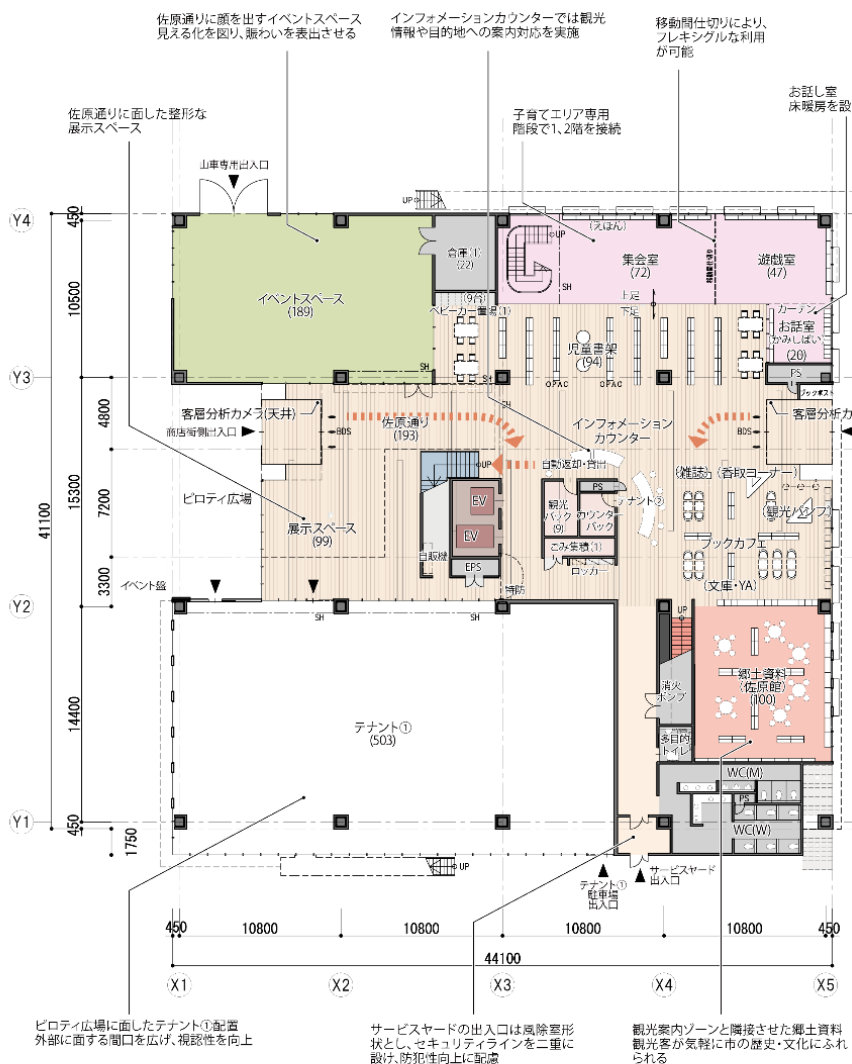
1階平面図
