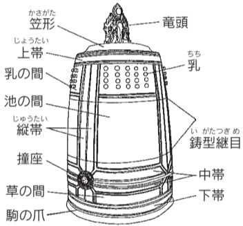
梵鐘各部の名称
